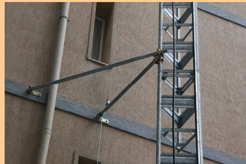
Detalle Anclaje
